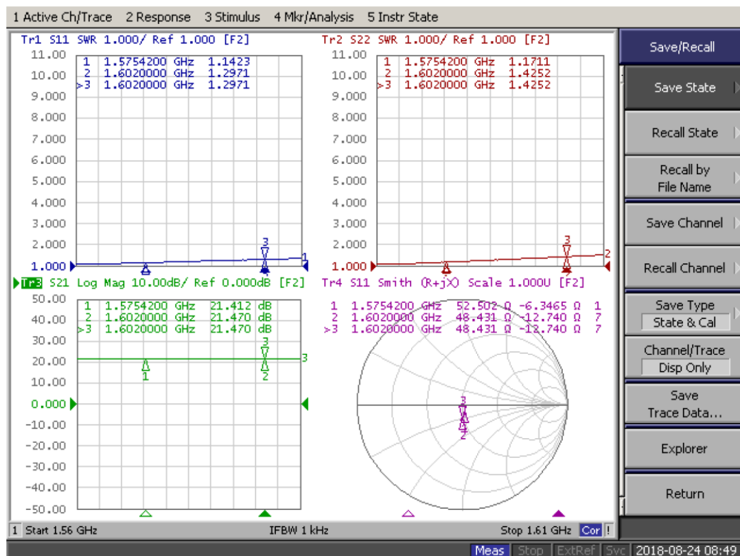
模块 RF 射频图:
